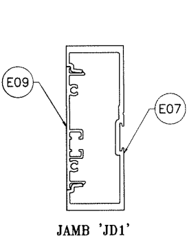
JAMB 'JD1'
